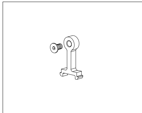
E56 ΣΥΝΔΕΣΜΟΣ ΧΩΡΙΣΜΑΤΟΣ ΑΛΟΥΜΙΝΙΟΥ ΓΙΑ ΠΡΟΦΙΛ (TV5 343) ALUMINIUM MULLION CONECTOR FOR PROFILE (TV5 343)
